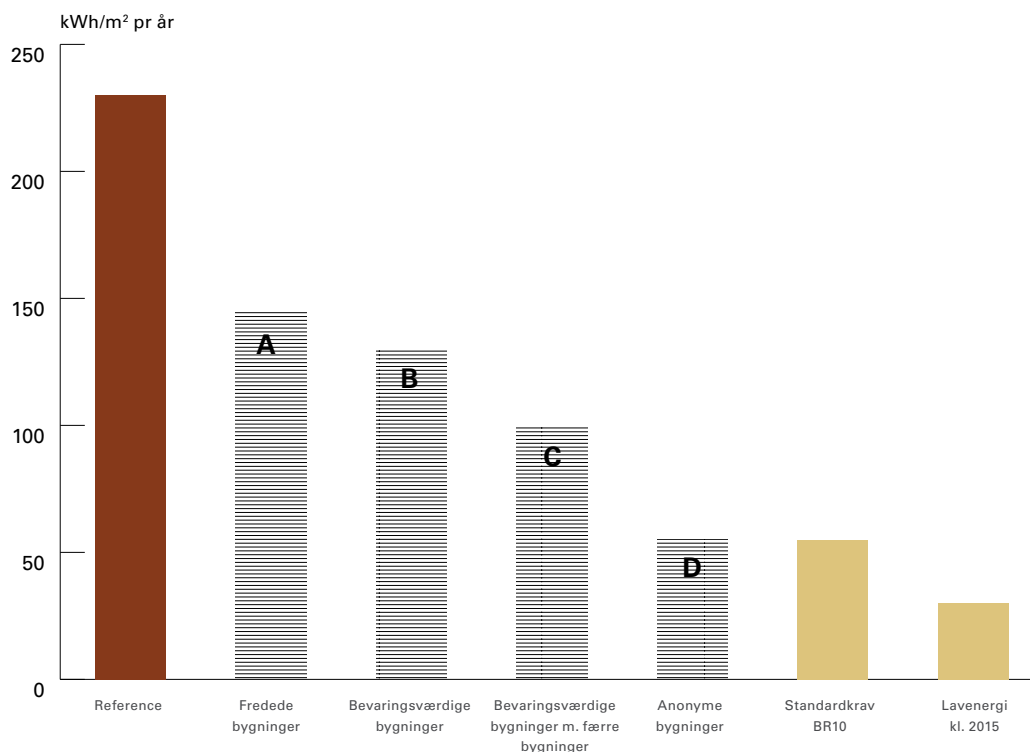
Figur 3. Energibehov for referenceejendom og ved energirenovering inden for de fire kulturarvskategorier.
