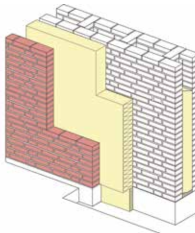
Figur 4. Udsnit i hulmur i tegl med faste bindere og udvendig efterisolering med ny skalmur.
